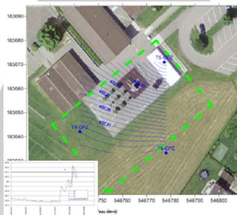
Isopièzes des eaux souterraines et variation des niveaux
