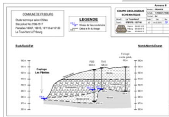
Hydrogeologisches Arbeitsmodell
